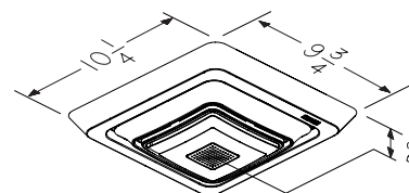
Dimensions illustrées en pouces.
